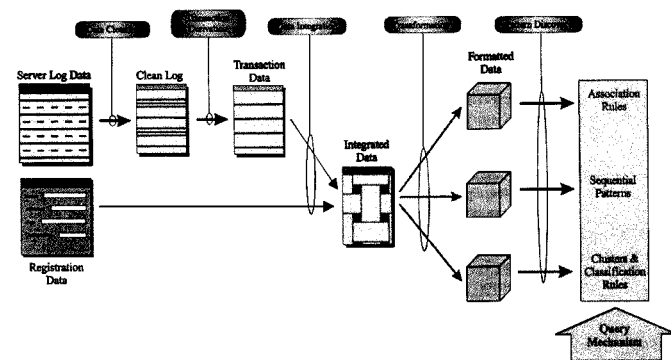
Fig. 4. Webminer architecture.
